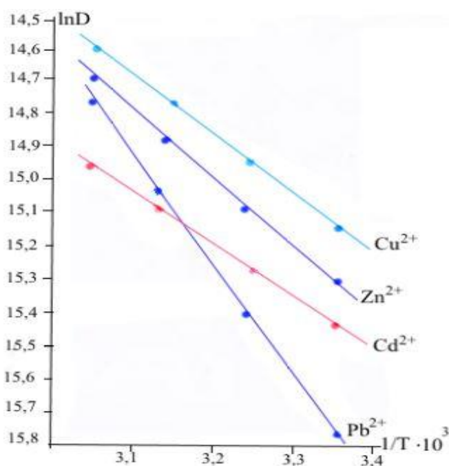
Şəkil 4. Öyrənilən ionların Amberlite MAC- 3 ioniti ilə udulmalarının temperaturdan asılılıq qrafikləri.
