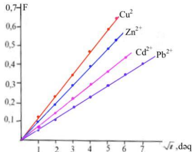
Şəkil 3. Öyrənilən ionların Amberlite MAC-3 ioniti ilə doyma dərəcəsinin t^{1/2} -dən
