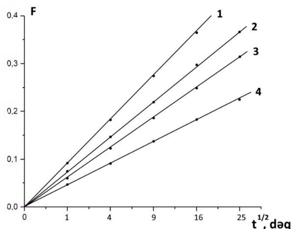
Şəkil 2. 2 sorbenti ilə Bi(III) ionlarının sorbsiyasının F-t^{1/2} asılılığı
