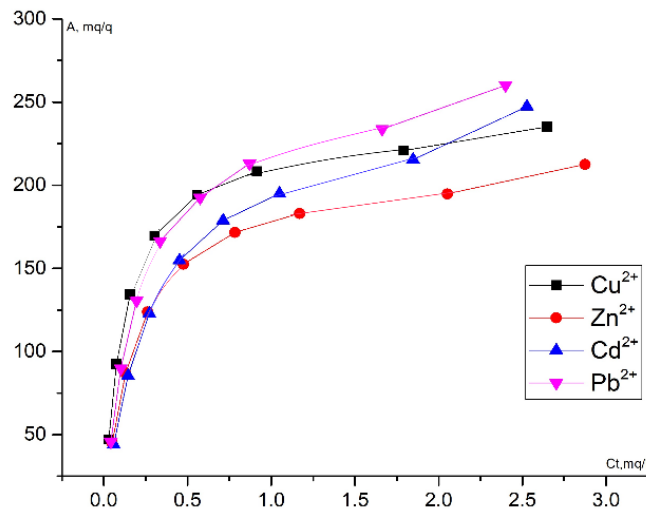
Şəkil 1. Öyrənilən Amberlite MAC-3 ioniti ilə Cu^{2+} , Zn^{2+} , Cd^{2+} və Pb^{2+} - ionlarının sorbsiya izotermələri.
