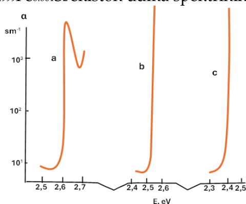
TlGa_{0.999}Fe_{0.001}S_2 ekiston udma spektrinin temperaturdan asılılığı
