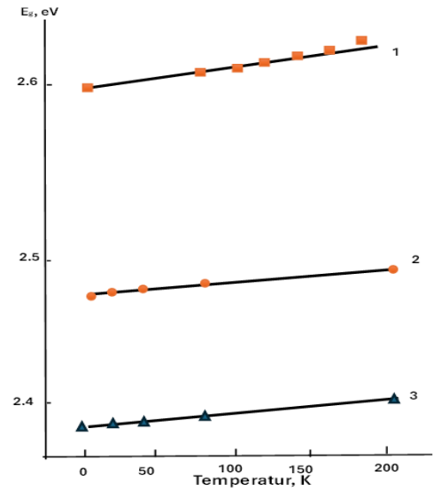
\text{TlGa}_{1-x}\text{Fe}_x\text{S}_2 kristalında E_g -nin temperaturdan asılılığı x=(1) 0, (2) 0.005, və (3) 0.01
