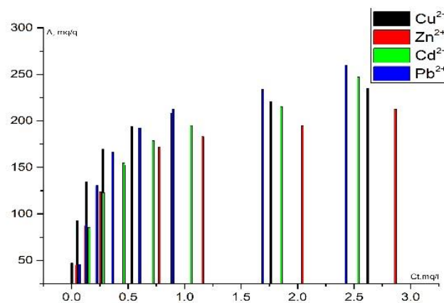
Şəkil 1. Öyrənilən Amberlite MAC-3 ioniti ilə Cu^{2+} , Zn^{2+} , Cd^{2+} və Pb^{2+} - ionlarının sorbsiya izotermələri.
