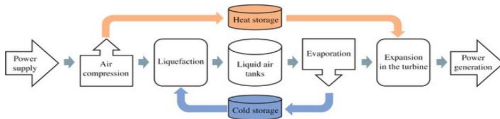
Şəkil 1. Maye havaya əsaslanan elektrik enerjisi saxlama qurğusunun iş prinsipinin sxemi.
