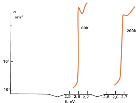
TlGa_{0.999}Fe_{0.001}S_2 ekiston udma spektrinin temperaturdan asılılığı
