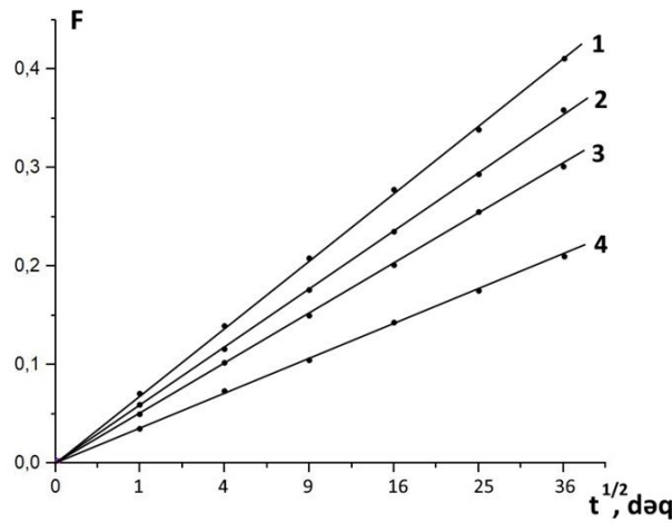
Şəkil 1.1 sorbenti ilə Cr(III) ionlarının sorbsiyanın F-t^{1/2} asılılığı
