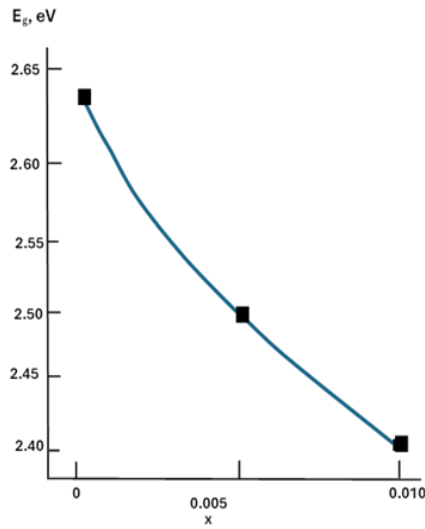
\text{TlGa}_{1-x}\text{Fe}_x\text{S}_2 kristalın 77K -də E_g -nin Fe konsentrasiyasından asılılığı
