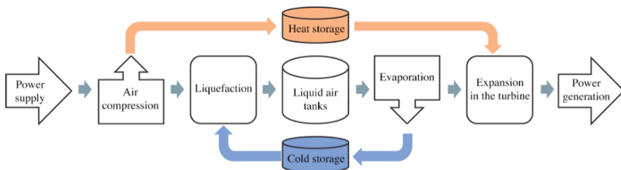
Şəkil 2. Maye havaya əsaslanan elektrik enerjisi saxlama qurğusunun iş prinsipinin sxemi
