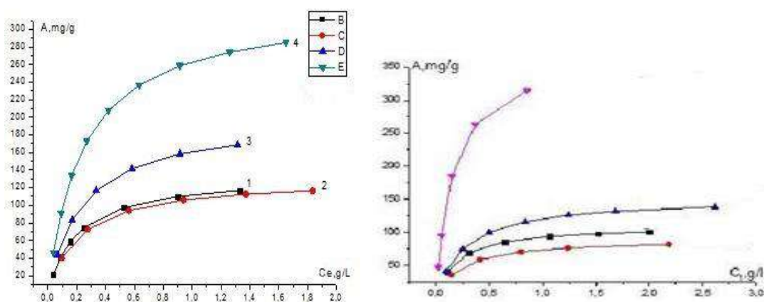
Şəkil 4. Diaion CR 11(sol), Purolite S 950(sağ) ilə öyrənilən ionların sorbsiya izotermələri: 1,2-Ag + ; 3-Zn 2+ ; 4-Cr 3+
