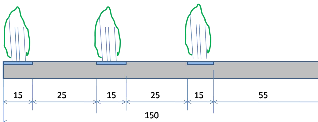
Şəkil 3 Tinglikdə səpin sxemi.
