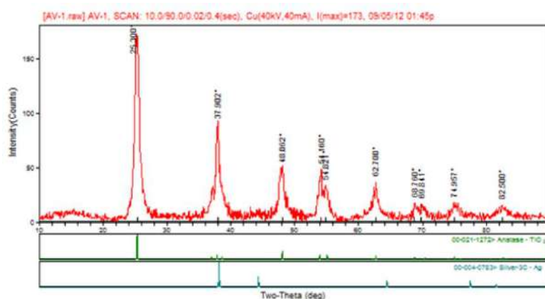
Şəkil 1. Sintez edilmiş F-1 nümunəsinin rentgen diffraktoqramı
