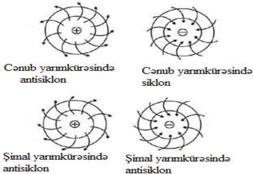
Şəkil 2. Siklon və antisiklon
