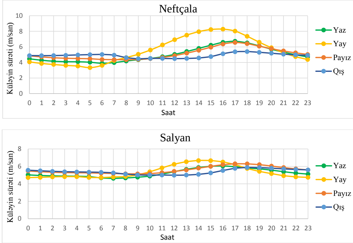
Şəkil 5. Salyan və Neftçalada külək sürətinin fəsillər üzrə günün müxtəlif saatlarında dəyişməsi
