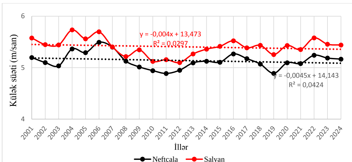
Şəkil 3. 2001-2024-cü illərdə Salyan və Neftçalada küləyin orta çoxillik sürətinin dəyişmə tendensiyası
