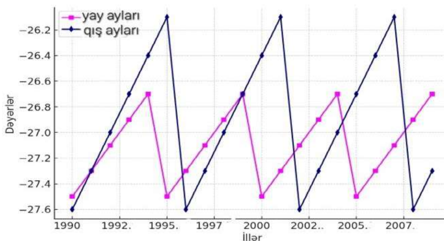
Şəkil 2. Xəzər dənizinin illərə görə səviyyəsi
