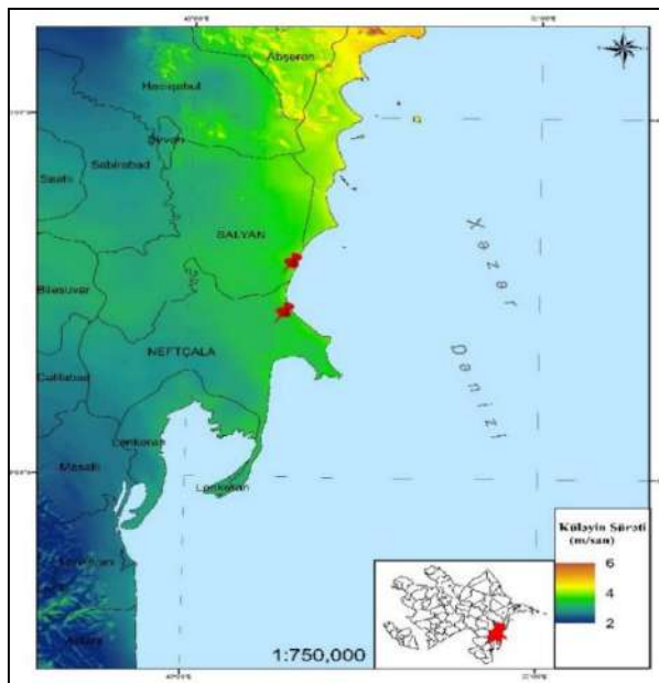
Şəkil 1. Tədqiqat nöqtələrində külək sürətinin xəritəsi [9]
