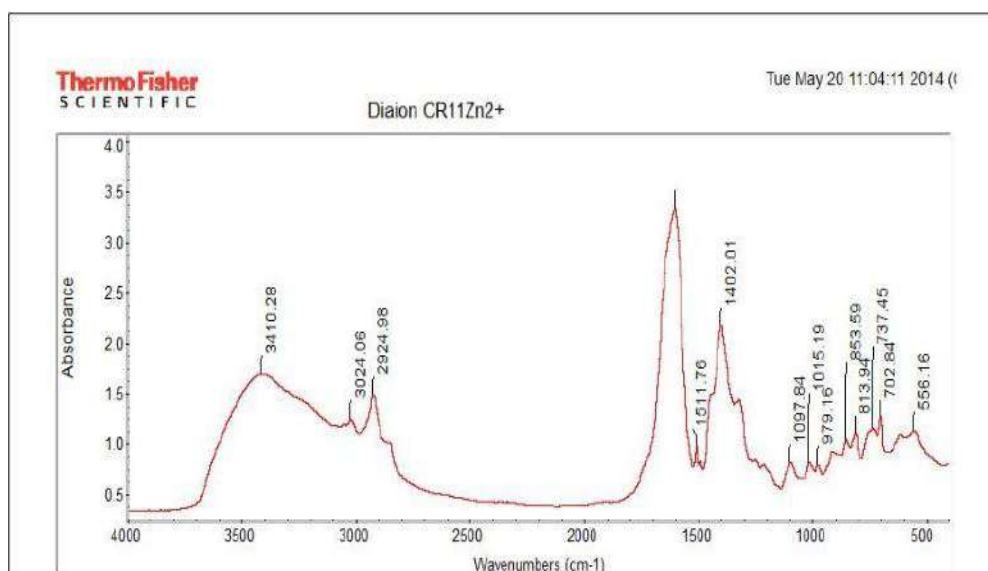
Şəkil 3. Diaion CR 11-in Zn^{2+} -ionları ilə işlənmiş formasının İQ-spektri
