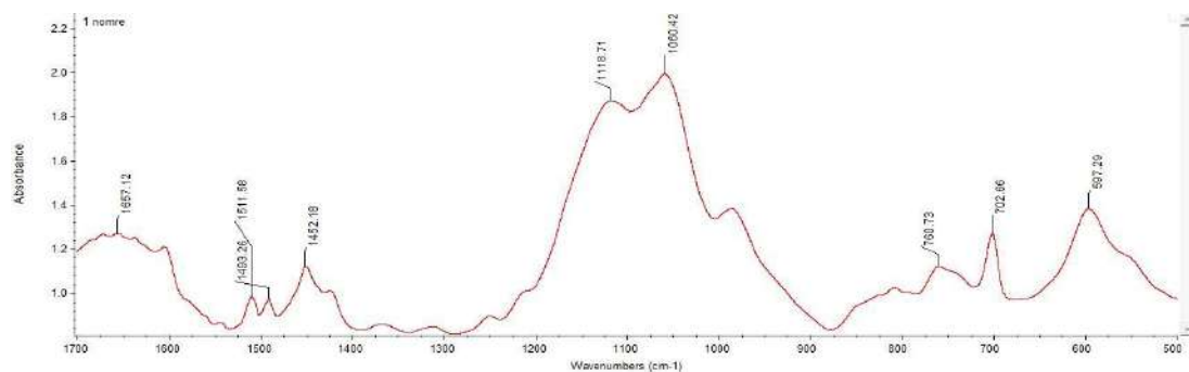
Şəkil 1. Purolite S 950(1) və onun Zn^{2+} (2), Cr^{3+} (3)-ionları ilə işlənmiş nümunələrinin İQ-spekləri
