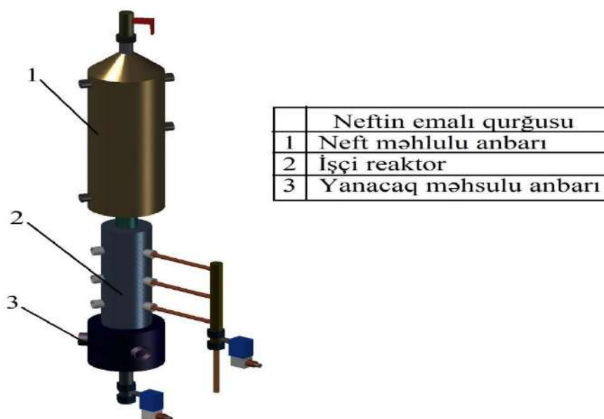
Şəkil 1. Neftdən yanacaq alınma qurğusunun sxemi
