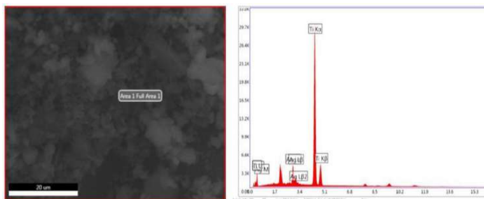
Şəkil 3. F-1 nümunəsinin EDS qrafiki
