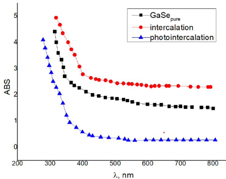
Şəkil 1. Udulmanın dalğa uzunluğundan asılılığı
