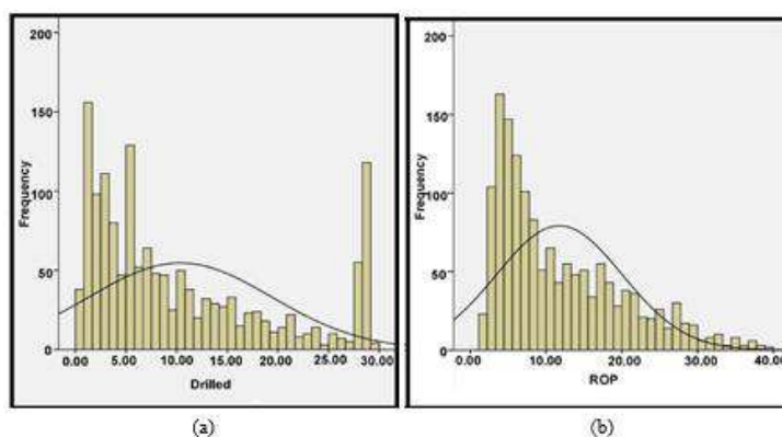
Şəkil 1. Qazma parametrlərinin normal əyrisi və histoqramı. (a) Qazılmış; (b) ROP(Qazma sürəti).
