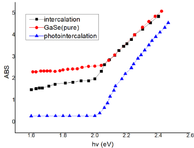
Şəkil 2. Udulmanın enerjidən asılılığı
