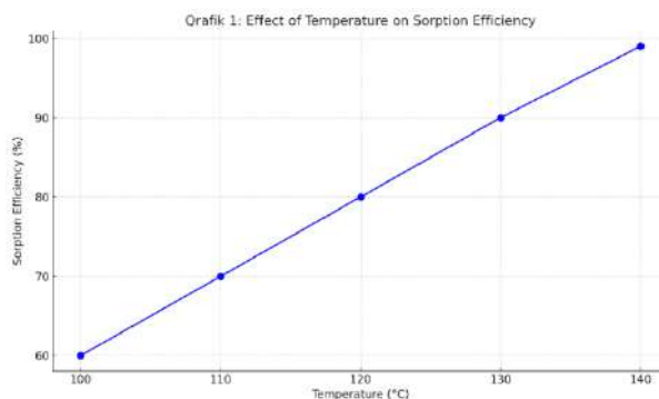
Qrafik 1 Temperaturun sorbsiya effektivliyinə təsiri, sorbsiya effektivliyinin 100°C-dən 140°C-yə qədər artan temperaturla necə yüksəldiyini göstərir.
