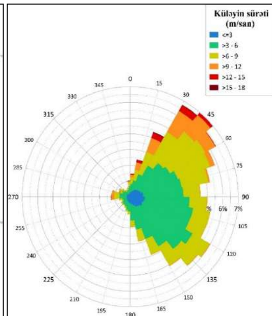
Şəkil 2. 2001-2024-cü illər üzrə Neftçala və Salyan üçün "külək gülü" qrafiki
