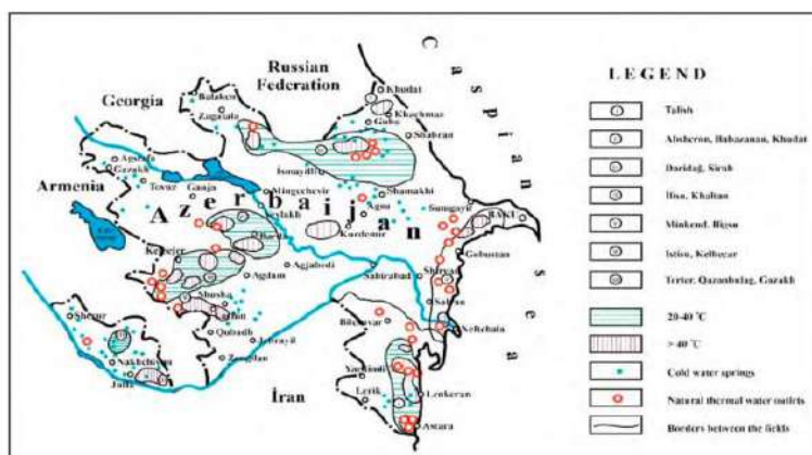
Şəkil 1. Azərbaycanda Termal su yataqları mənbələrinin sxematik xəritəsi
