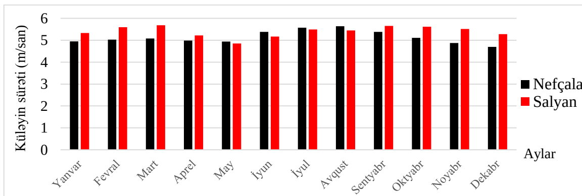
Şəkil 4. Salyan və Neftçala üzrə küləyin orta aylıq sürət qrafiki
