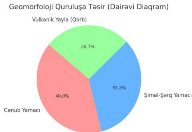
Diaqram 2. Kiçik Qafqaz ərazisində ekocoğrafi komponentlərin geomorfoloji quruluş təsir dərəcəsi
