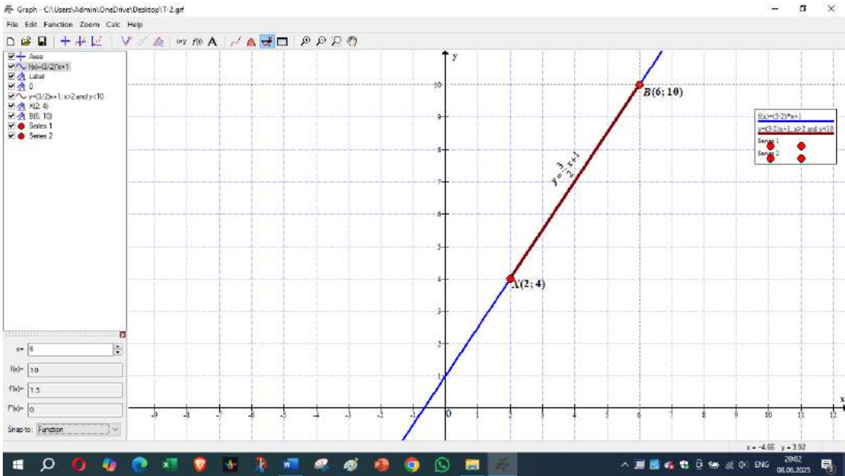
Şəkil 2. X(2; 4) və B(6; 10) nöqtələrindən keçən düz xəttin qrafiki
